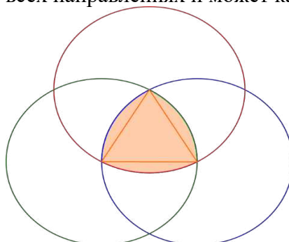
Рисунок 2 - Треугольник Рёло
