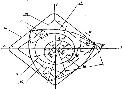
Рисунок 5 - Образование гипоциклоид
