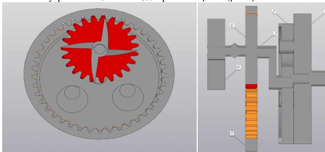
Рисунок 4 - 3D модель циклоидального привода с рабочими органами по принципу Треугольника Рёло
